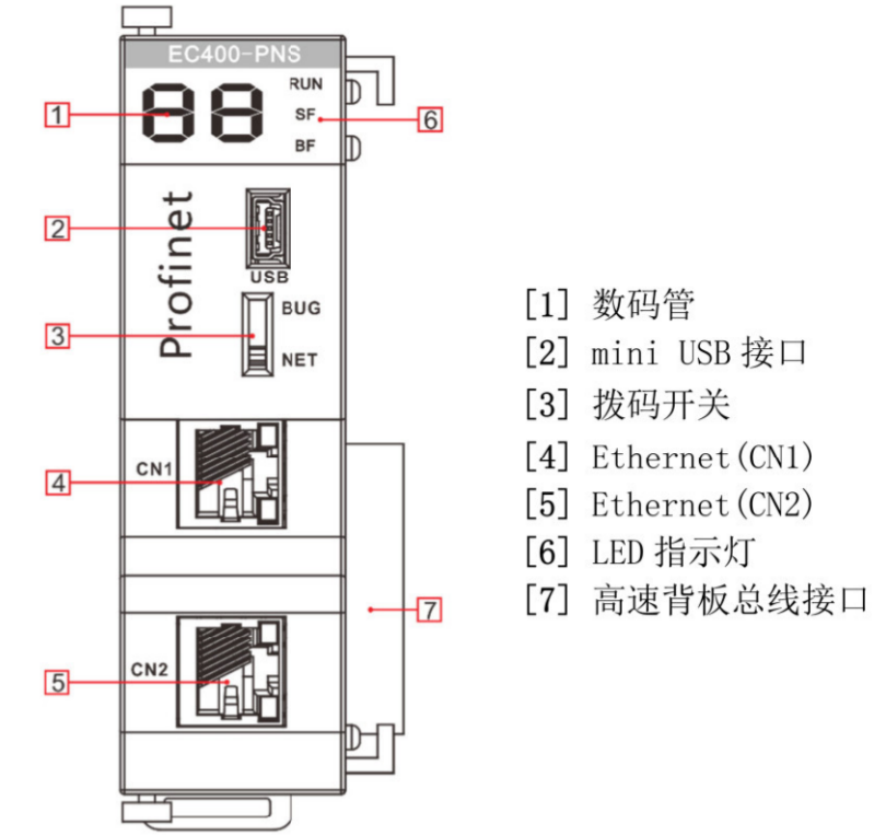
图 2 EC400-PNS 模块接口示意图
