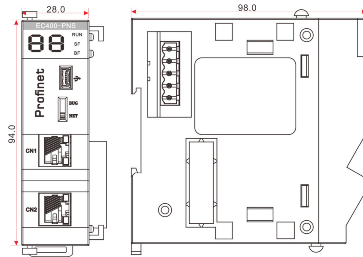
图 1 EC400-PNS 机械尺寸 (单位: mm)
